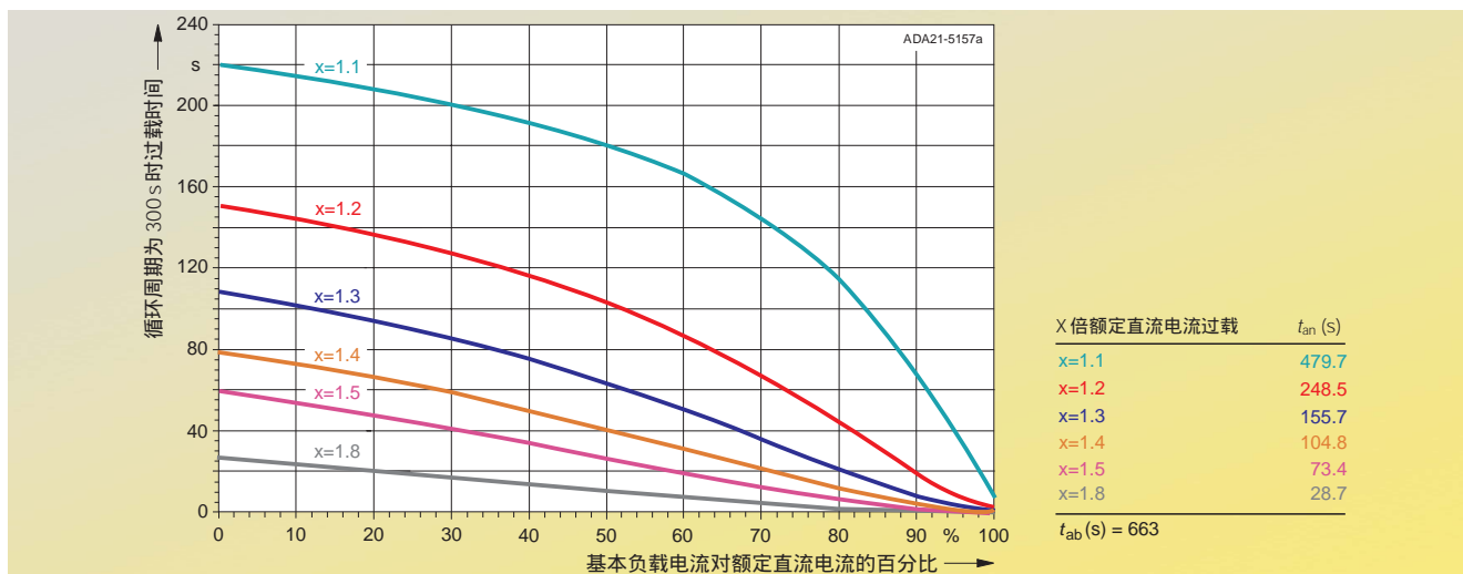
图 5/29 6RA7095-4KS22 2000 A / 1Q / 690 V
