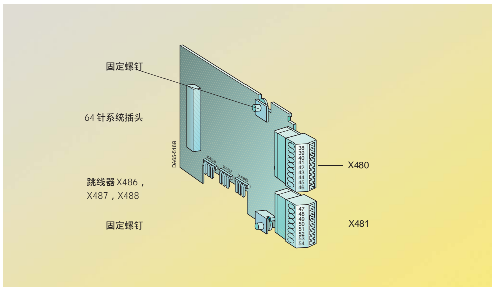
图 4/10 端子扩展板 EB1
