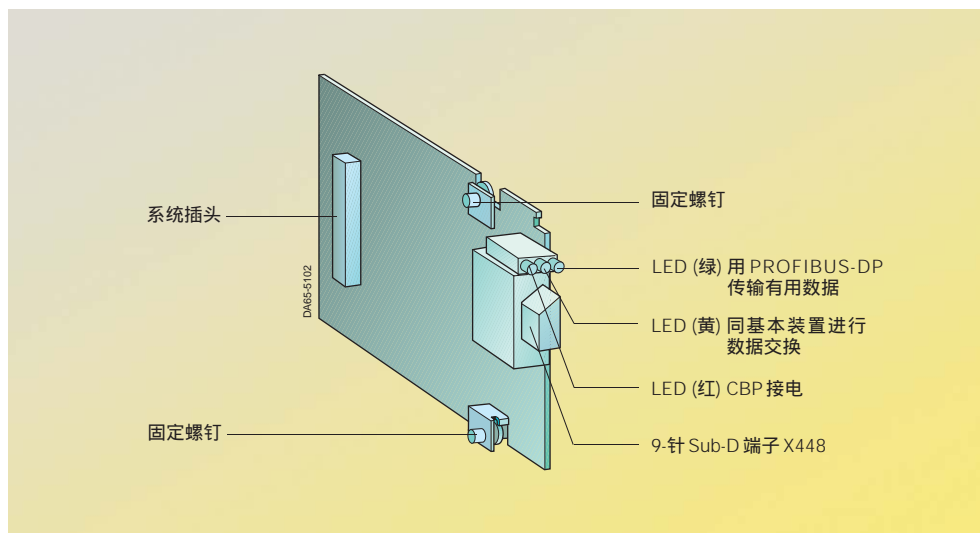
图 4/21 通讯板 CBP2
