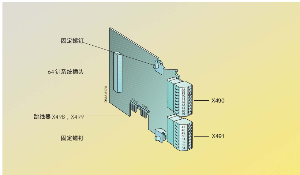
图 4/12 端子扩展板 EB2
