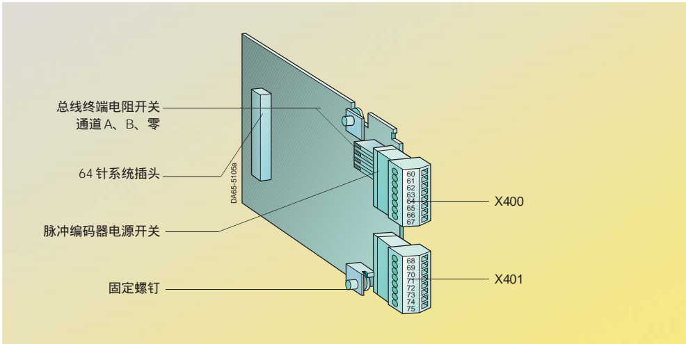
图 4/9 选件板 SBP
