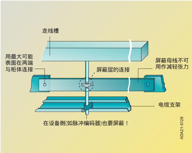
图 5/37 电缆进入柜体处的屏蔽连接
