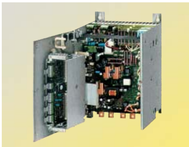
图 2/2 SIMOREG 6RA70, 15 A/30 A
