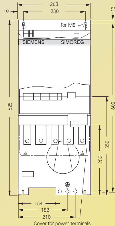
图 2/11 额定电流 400-600 A 的 SIMOREG K 6RA28 整流装置
