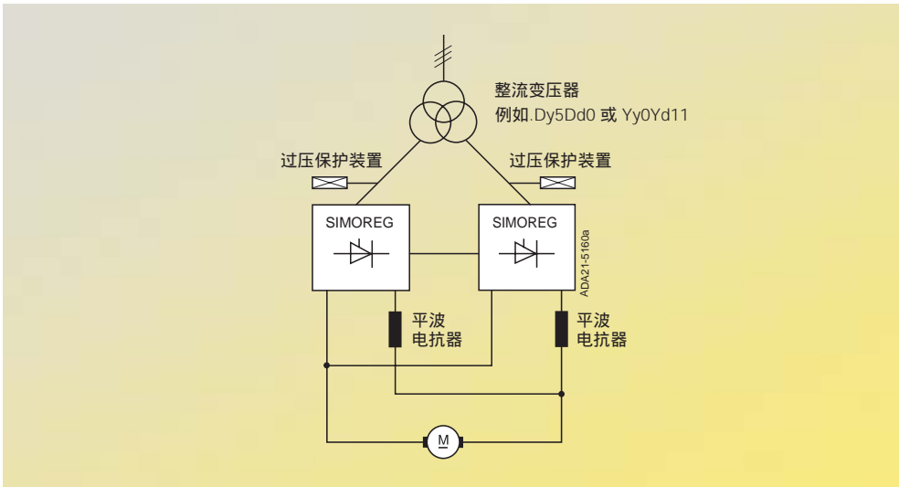
图 5/35 12 脉动传动系统
