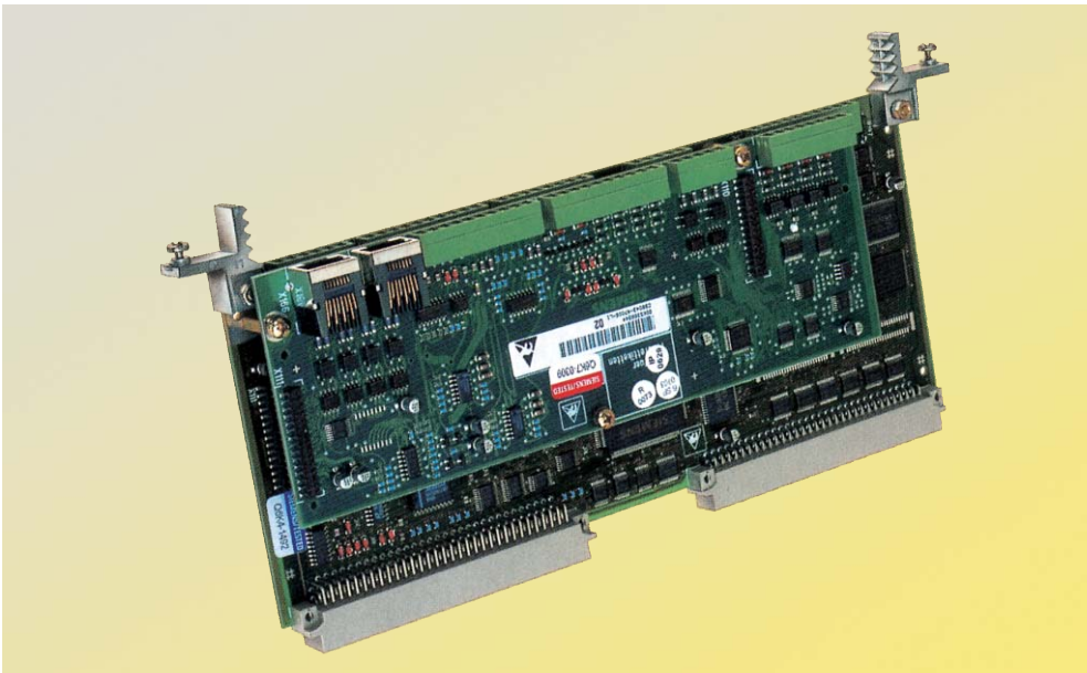
图 4/2 端子扩展板 CUD2 插在基本电子板 CUD1 上
