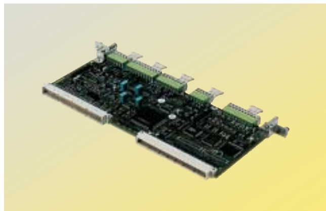
图 2/1 基本电子板
