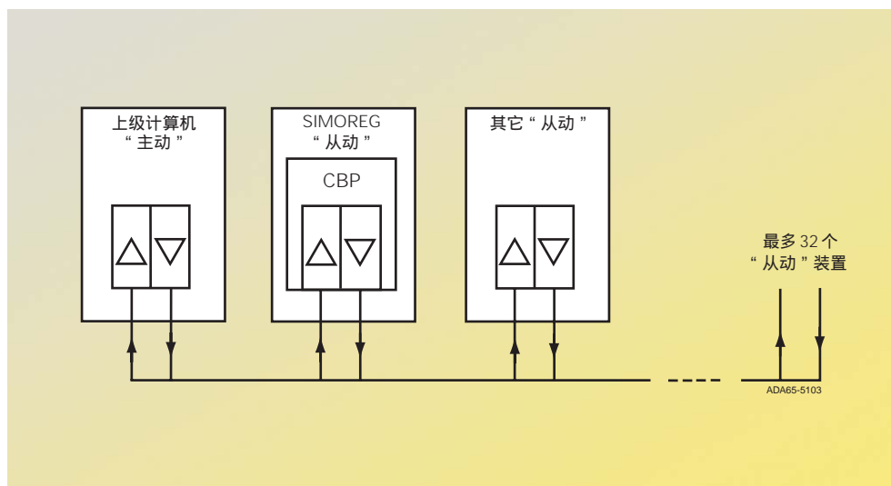
图 4/22 PROFIBUS-DP 连接
