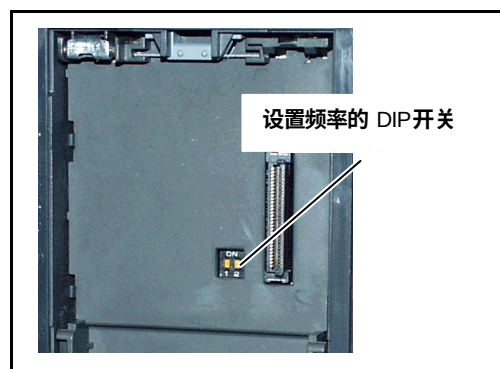
图 3-4 DIP 开关
