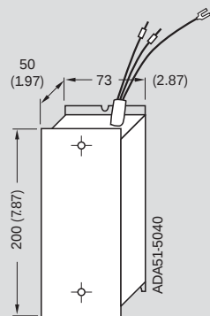
背板式安装的进线电抗器
