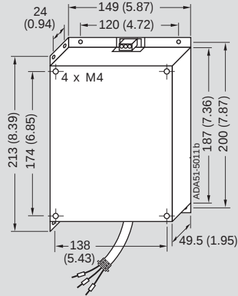
适合 B 型外形尺寸变频器的滤波器
