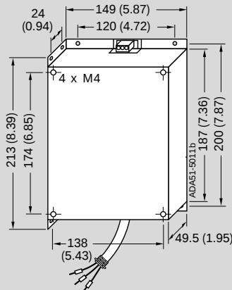
适合 B 型箱体尺寸的滤波器
