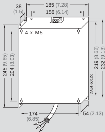
适合 C 型箱体尺寸的滤波器
