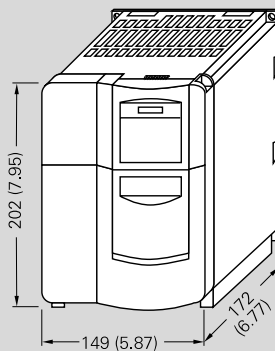
B 型箱体尺寸变频器
