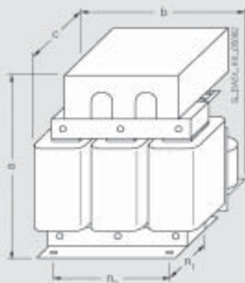
落地式安装，M10 螺栓 D 至 F 型变频器适用的 LC 滤波器
