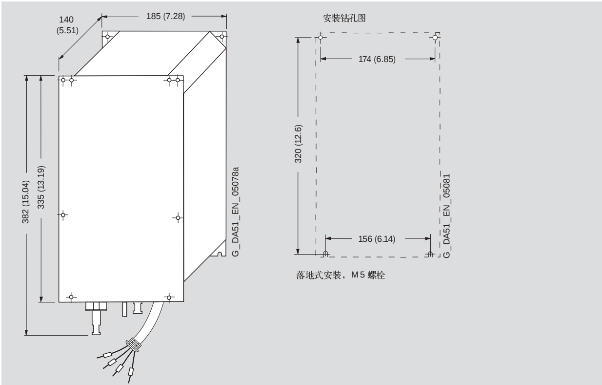
C 型变频器适用的 LC 滤波器
