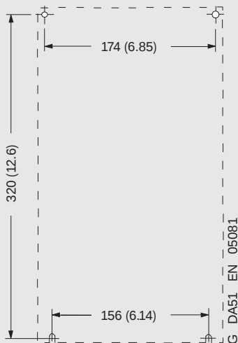
落地式安装，M5 螺栓
