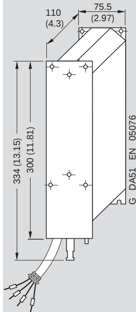
A 型变频器适用的 LC 滤波器
