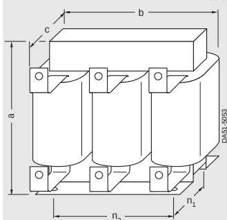
适合 FX 和 GX 型外形尺寸变频器的进线电抗器
