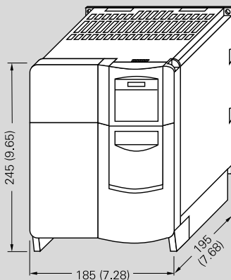
C 型箱体尺寸变频器
