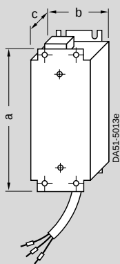
适合 A 型箱体尺寸 的进线电抗器
