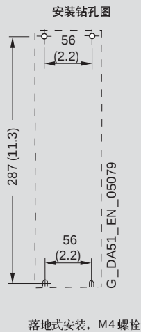
落地式安装, M4 螺栓
