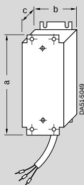
适合 A 型箱体尺寸的输出电抗器
