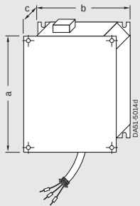
适合 C 型外形尺寸变频器 (电源电压为 500-600V, 3AC) 的进线电抗器
