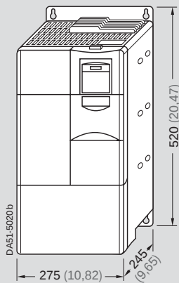
D 型外形尺寸的变频器
